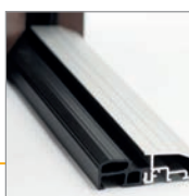
Próg aluminiowy z przekładką termiczną
