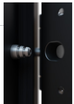
3 bolce przeciwwyważeniowe
