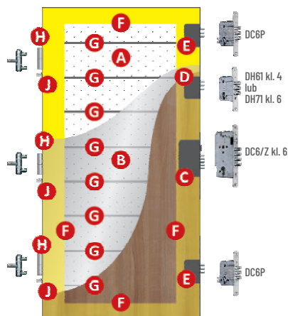
Budowa skrzydła drzwiowego
