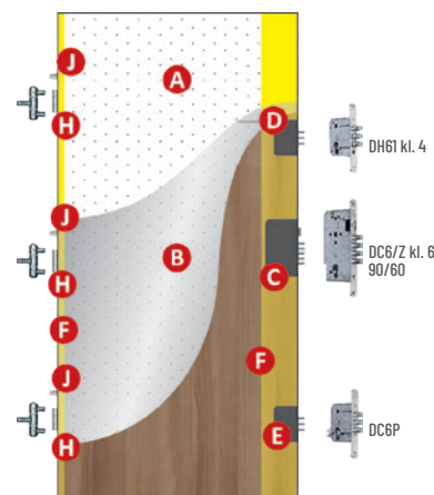
Budowa skrzydła drzwiowego
