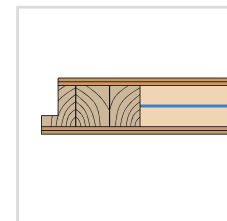
SKRZYDŁO 46 mm wzmocnione blachą stalową
